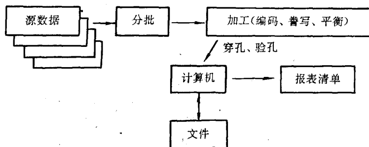
(a) 文件批处理
