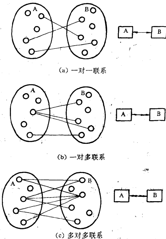
图 1-8 总体之间的联系方式
