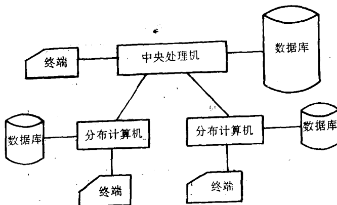
(c) 分布式处理
