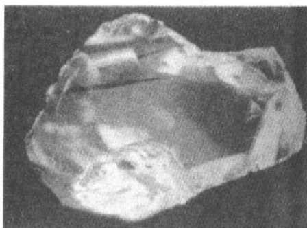
图 1.4 金刚石晶体在阴极射线中发光 [3]
