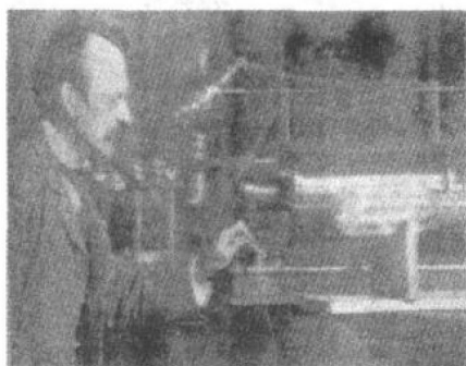
图 1.3 汤姆逊发现电子 [3]
