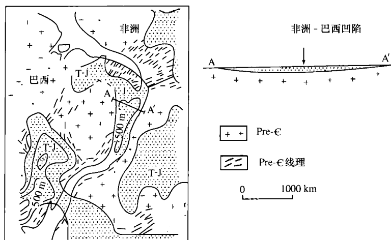
图 1-8 克拉通内部的古地理
