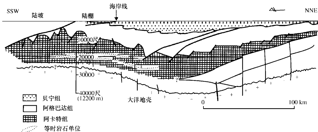
图 1-7 尼日尔三角洲沉积剖面图
