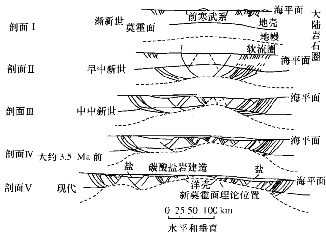
图 1-6 南红海的构造演化系列
