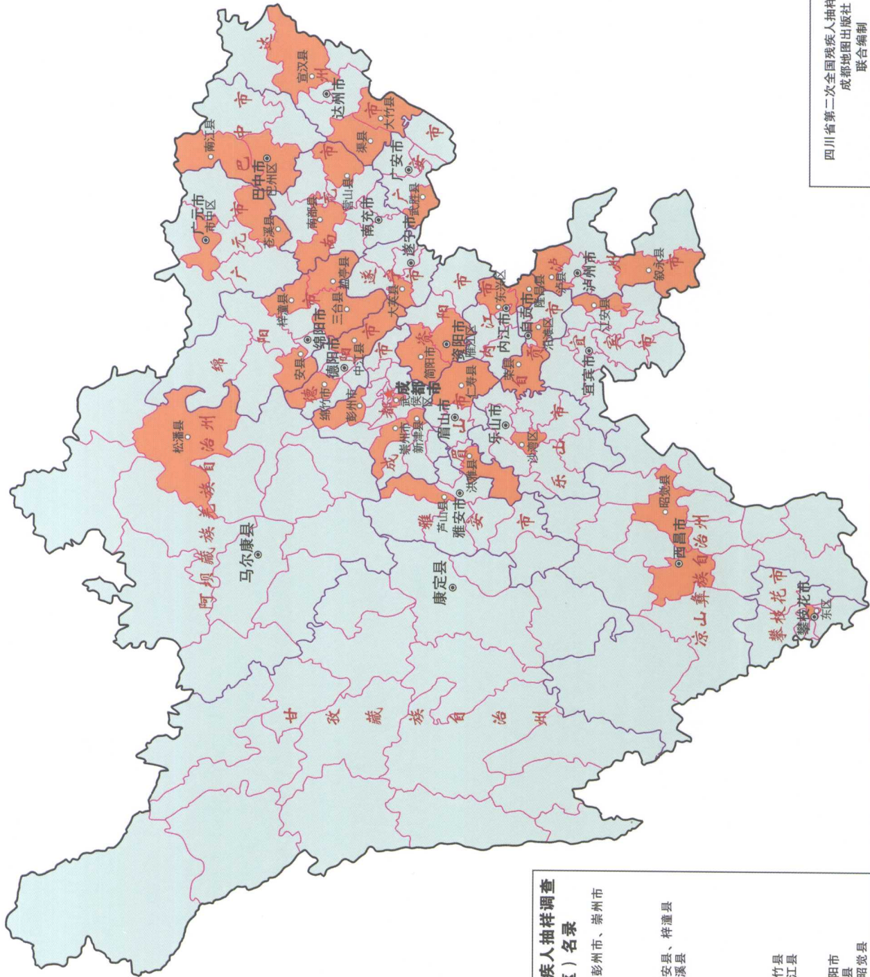
四川省第二次全国残疾人抽样调查样本县(市、区)分布示意图
