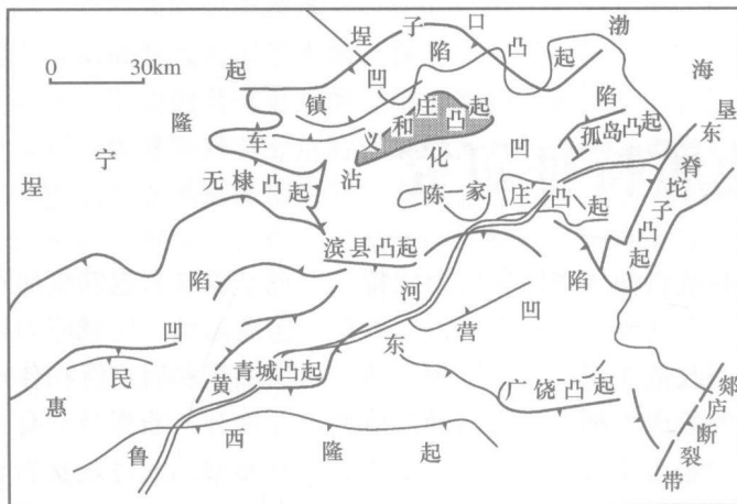
图 2-1 济阳坳陷地质结构略图
