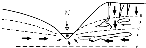
图 2-3 岩溶水动力垂直分带示意图
