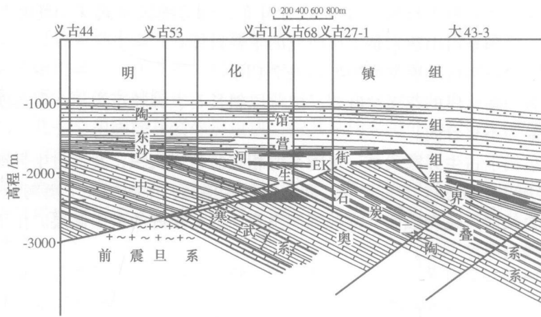
图 2-2 屋脊式潜山断块油藏剖面图
