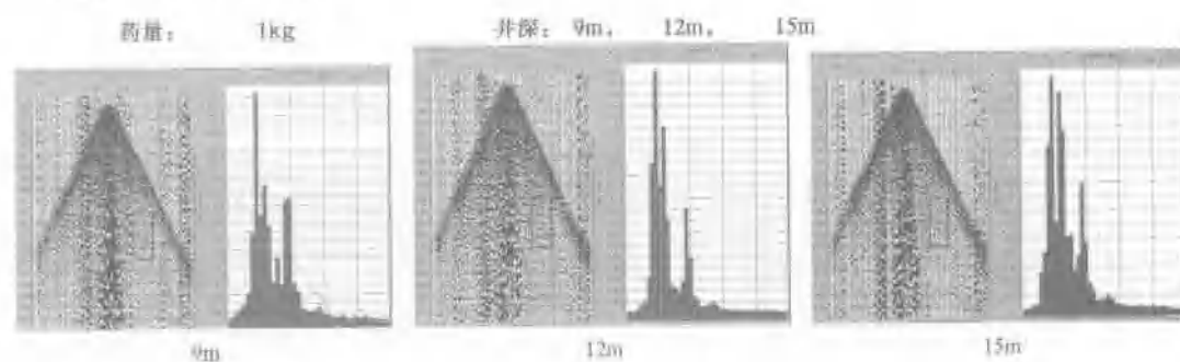
图 1-3-1 井深试验频谱分析图
