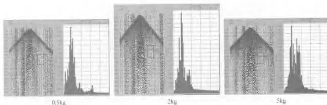
图 1-3-2 药量试验频谱分析图
