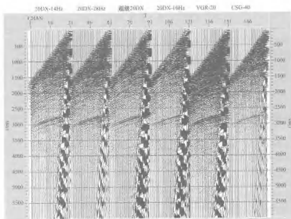
图 1-3-3 检波器对比记录
