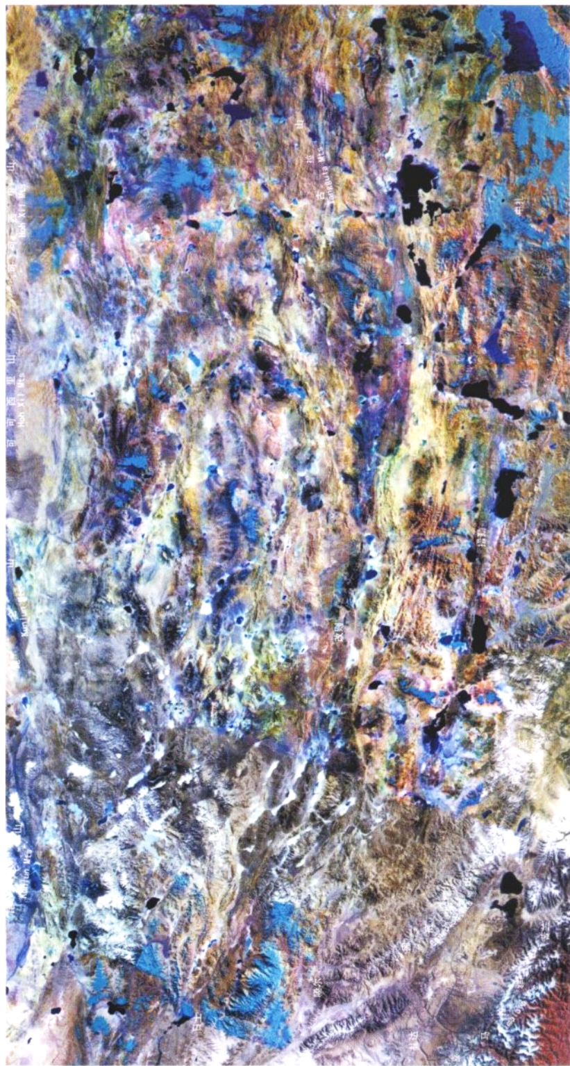
西藏羌塘地区卫星遥感影像图
