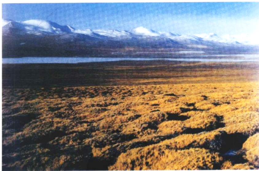
羌塘盆地南部坳陷区地貌
