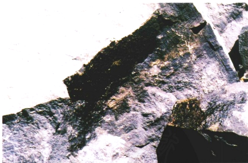
安多北114道班上侏罗统索瓦组灰岩中的液态油苗
