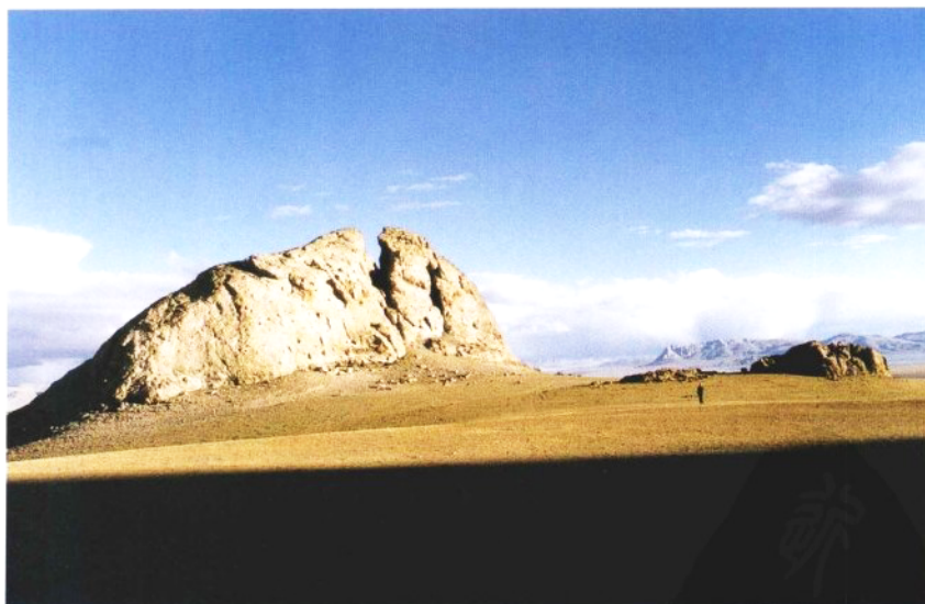
羌塘盆地中侏罗统中的点礁
