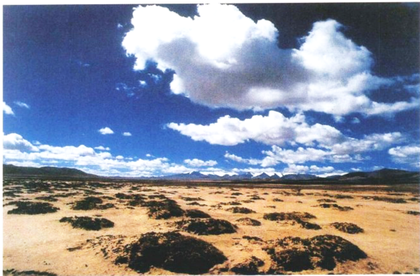
羌塘盆地北部坳陷区地貌
