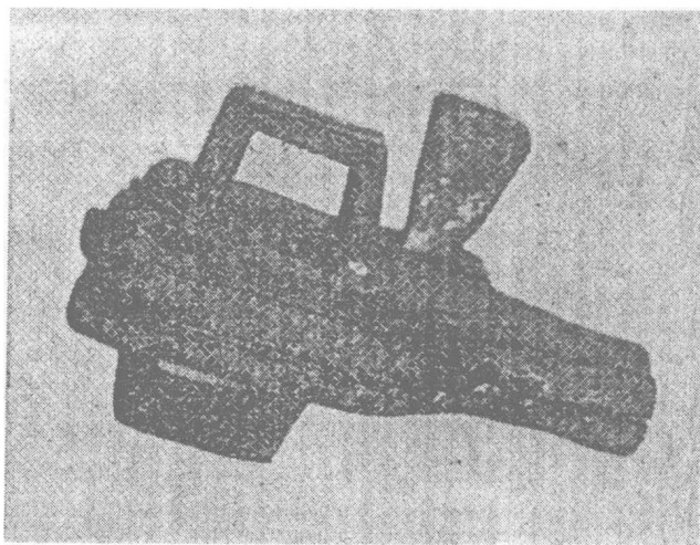
河北兴隆（热河）发现战国时期的燕国冶铁遗址制造锄具的铁范
