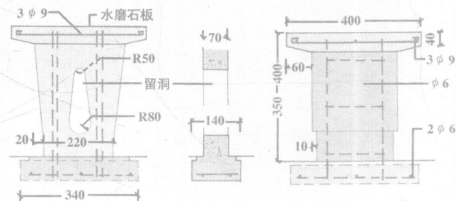
5. 钢筋混凝土条凳构造
