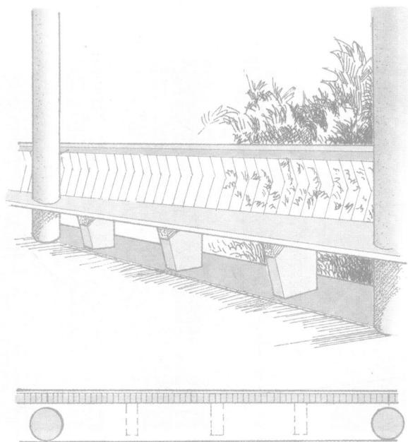
10 钢筋混凝土靠背坐椅构造(2)
