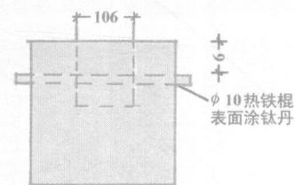
底脚正剖面
