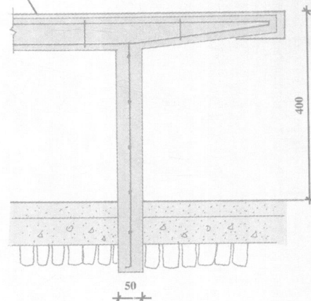
2-2 剖面
