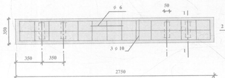
2. 钢筋混凝土坐凳构造
