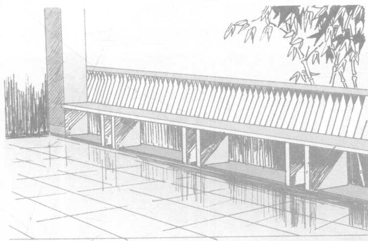
3. 钢筋混凝土靠背椅构造(1)
