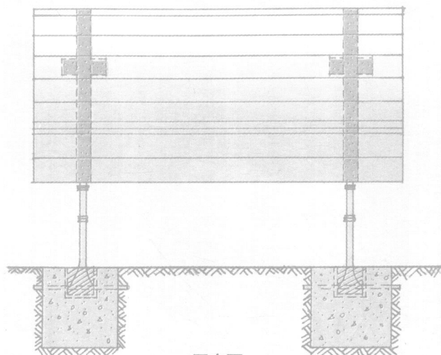
正立面
