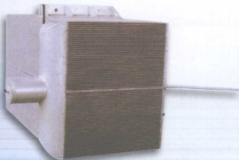
△ 冷凝蒸发器 (6000m 3 /h 空分设备用)
