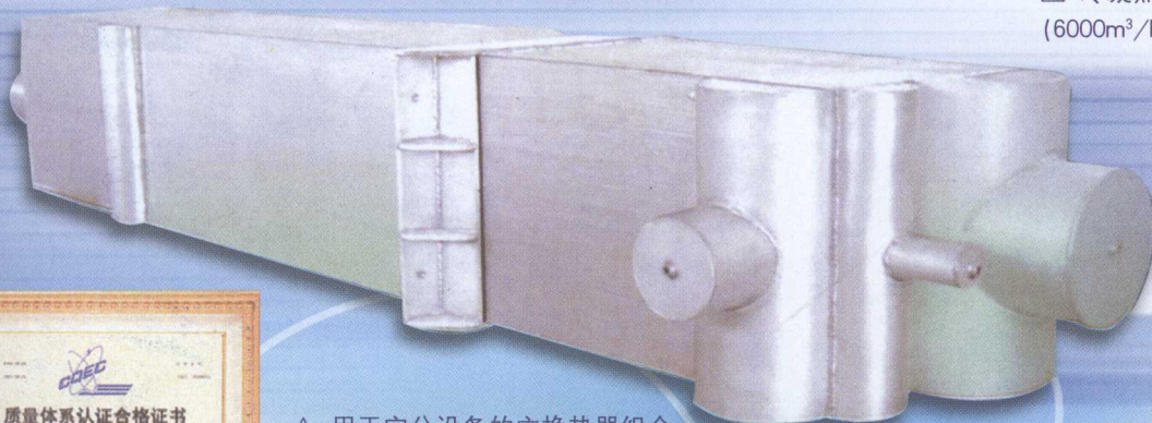
△ 用于空分设备的主换热器组合 (1100mm × 1100mm × 5700mm)
