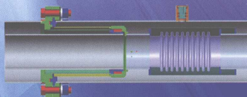
真空管道法兰连接结构简图
