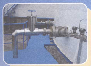
● 紧急切断阀
