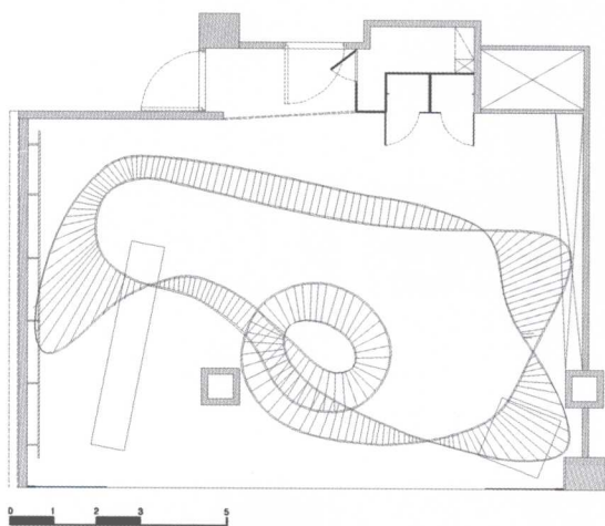
平面图
