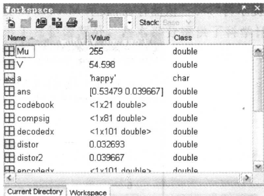
图 1-5 Workspace
