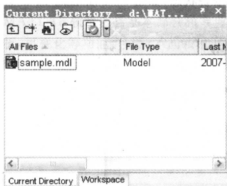
图 1-4 Current Directory
