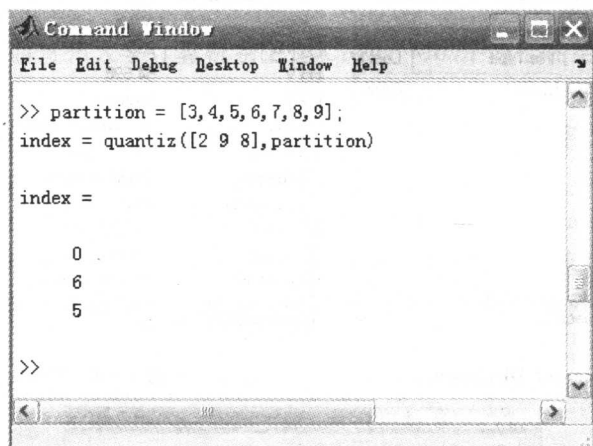
图 1-3 Command Window
