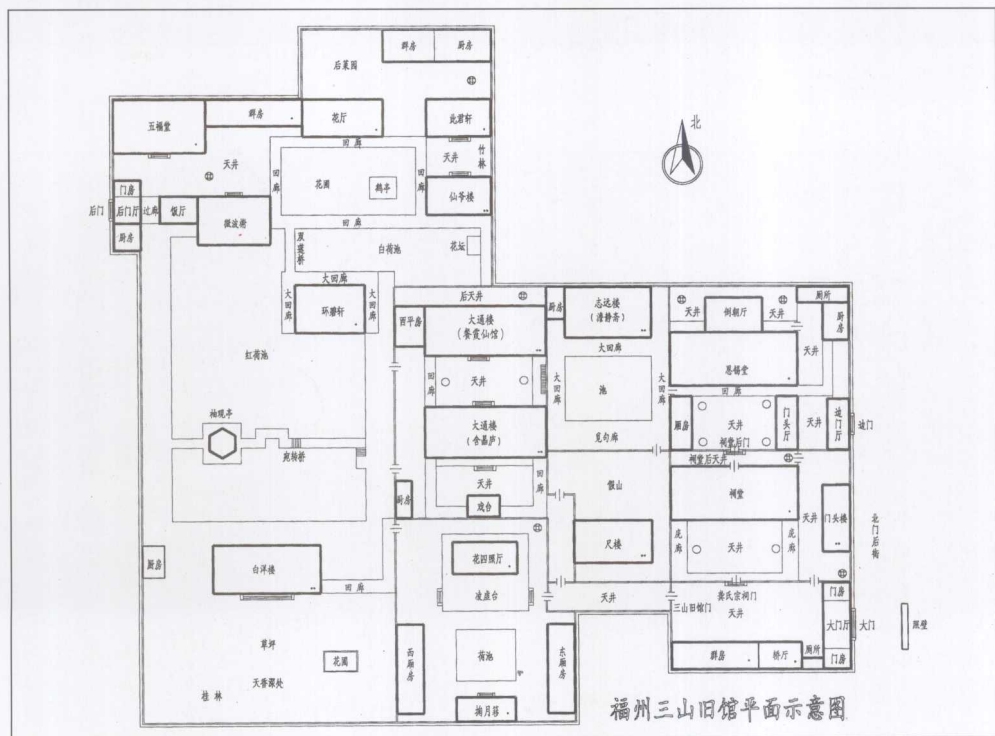
龚易图的“三山旧馆”平面图
