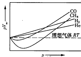
图 1.1 几种气体的 pV_m - p
