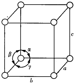
图 1.2 晶胞参数
