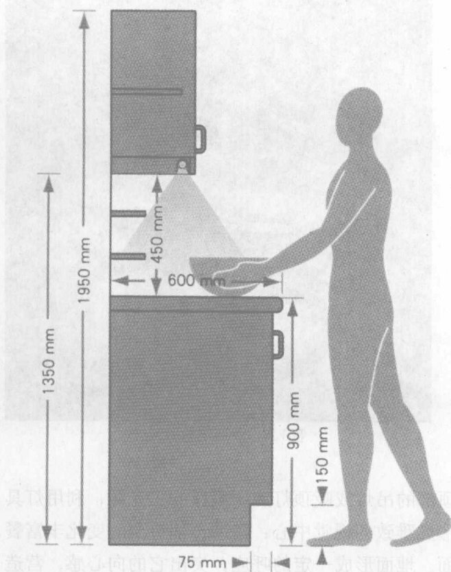
图1.6 厨房操作台面尺度
