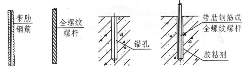
图1.2 化学植筋
