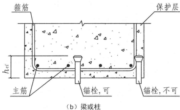
图4.9 锚栓位置要求
