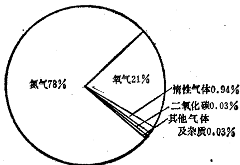
图 1-1 空气的组成
