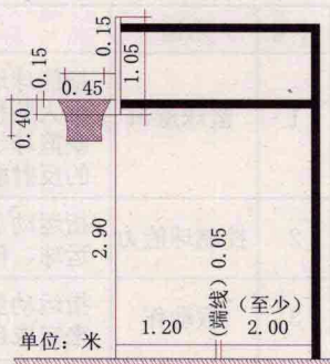
图1-1-3 球篮与篮板的尺寸
