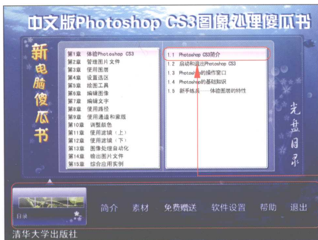
图1 光盘主界面
