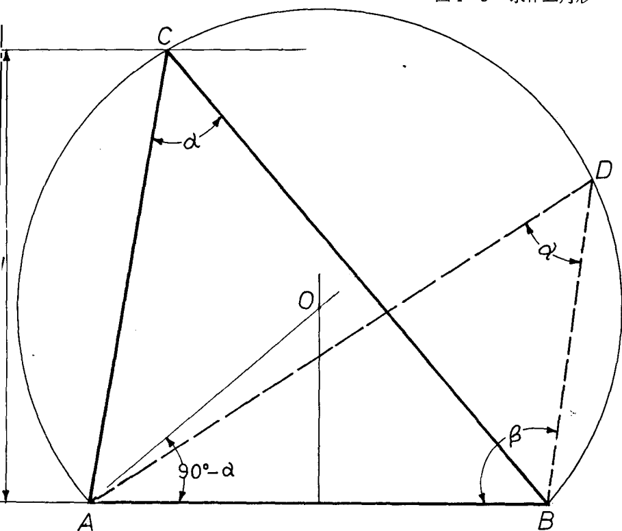
圖 1-3 求作三角形
