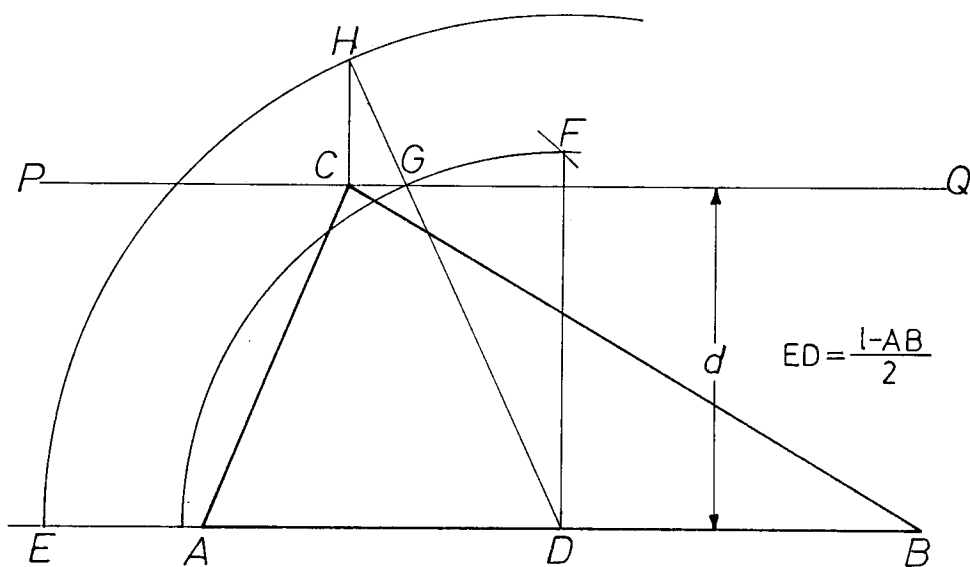
圖 1-6 求作三角形
