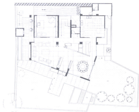
一楼平面配置图
