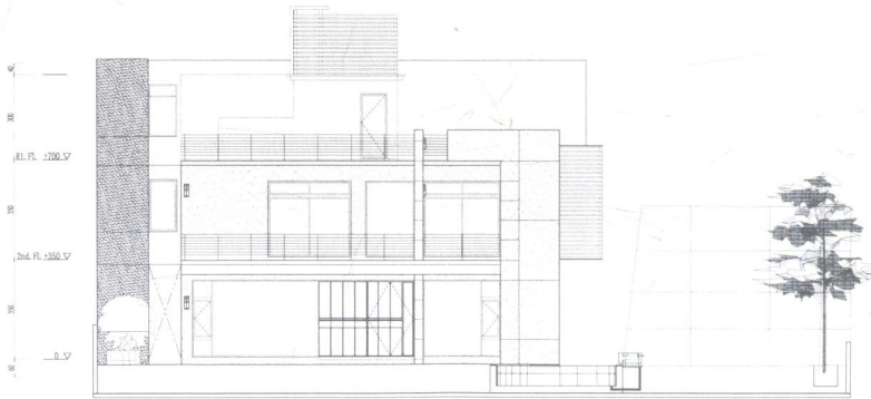
西侧外观立面图
