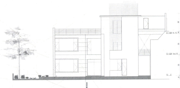
北侧外观立面图
