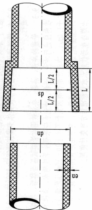
粘接连接承插口
