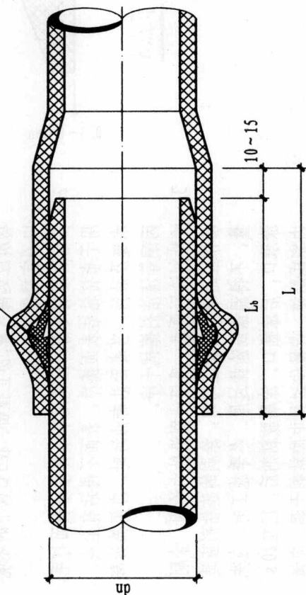
橡胶密封圈
