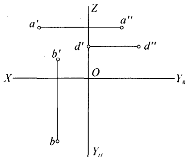
(a) 已知条件
