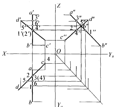
(b) 作图过程
