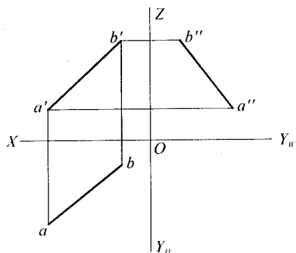
(a) 已知条件
