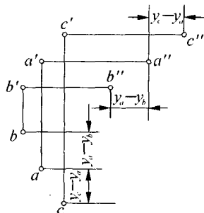
(c) 作图过程(二)
