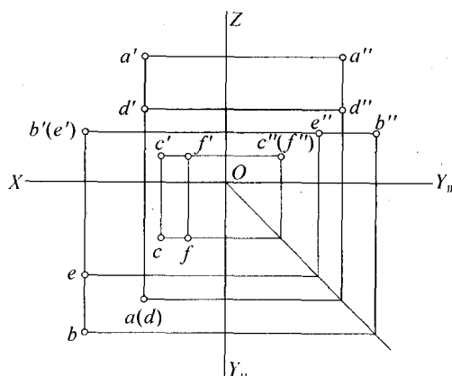
(b) 作图过程
