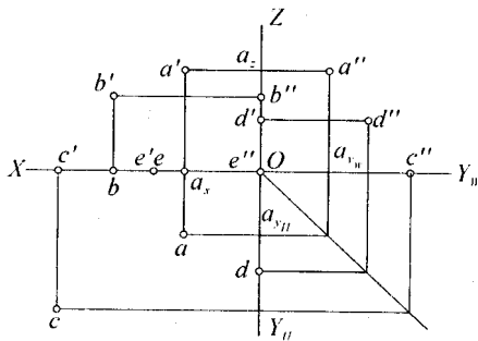
(b) 作图过程
