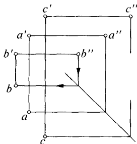
(b) 作图过程(一)
