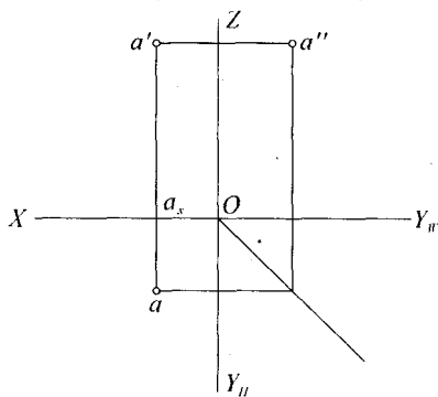
(a) 已知条件
