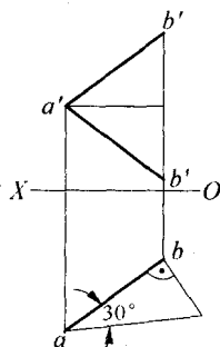
(b) 作图过程
