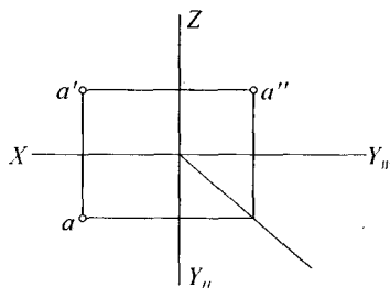
(b) 作图过程
