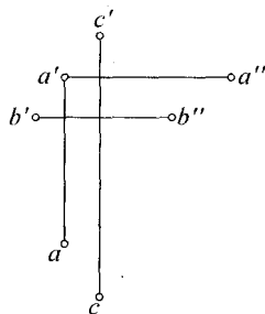
(a) 已知条件
