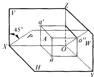
(a) 空间状况分析
