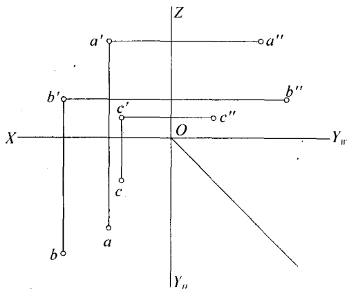
(a) 已知条件
