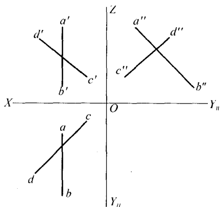
(a) 已知条件
