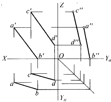
(b) 作图过程
