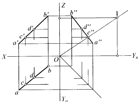
(b) 作图过程
