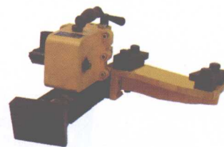
液压方枕器
