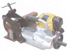
DUBUIS四冲程内燃钻孔机
