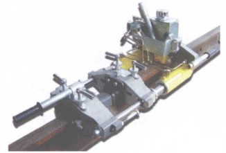
钢轨除瘤机EPM2整体式
