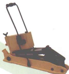
液压拨道器
