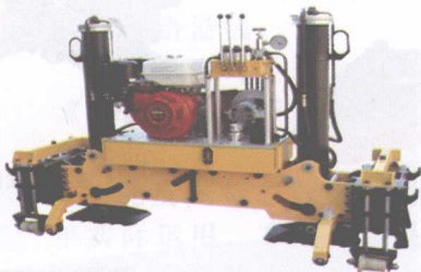
YQB-6.5 液压起拨道机
