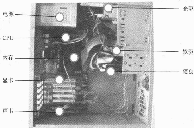
图 1-14 电脑的内部结构
