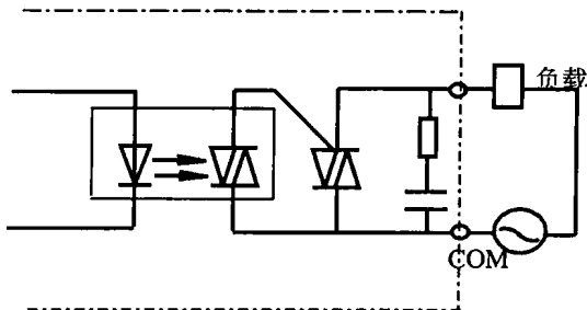
图 2-5 晶闸管输出电路
