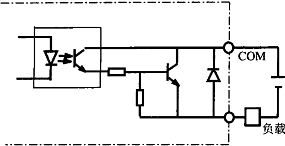
图 2-4 晶体管输出电路
