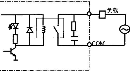
图 2-3 继电器输出电路
