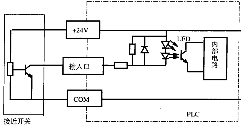
图 2-2 直流输入接线图
