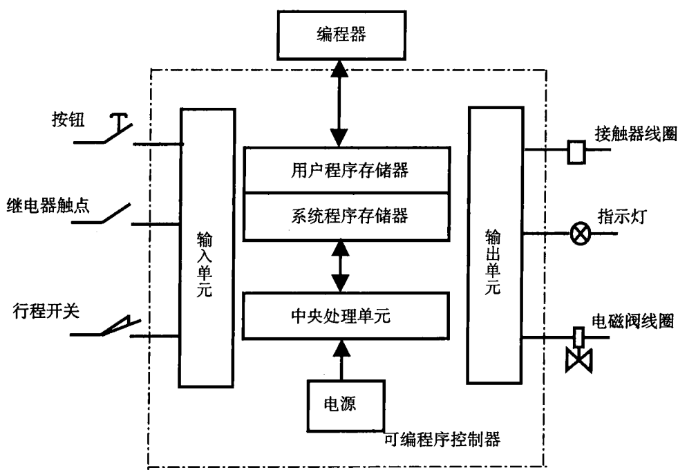
图 2-1 PLC 结构框图
