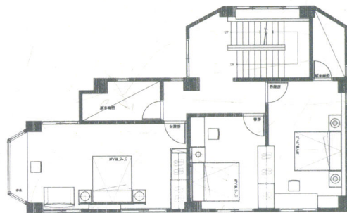
三楼平面配置图
