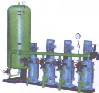
MCI 型自动稳压给(排)水成套设备
