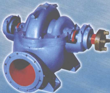
Sh 型单级双吸式离心泵
