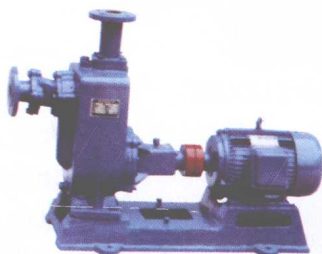
ZW 型自吸无堵塞排污泵
