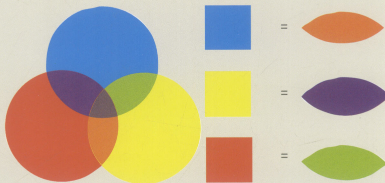
互补色图表
