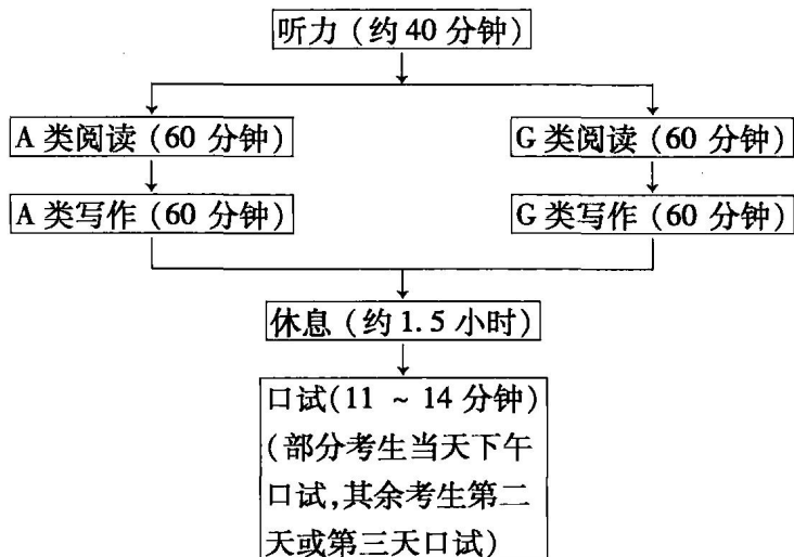
图 1 考试流程图
