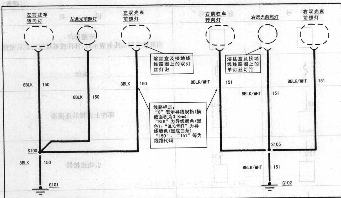
图 1-4 上海通用汽车电路图中的接地电路
