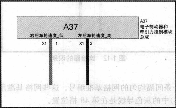
图 1-15 总成标识
