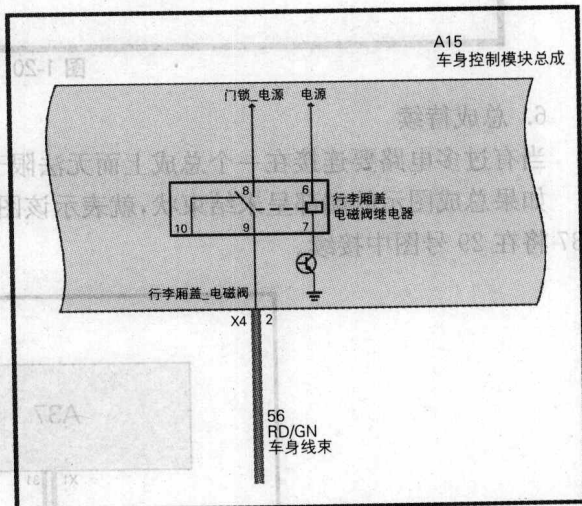
图 1-18 总成内的信息
