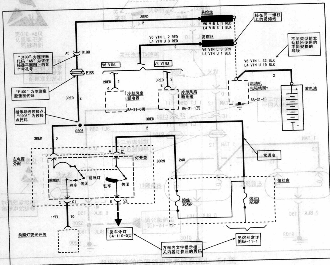
图 1-1 上海通用汽车电路图中的电源电路
