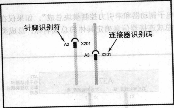
图 1-12 连接器的识别
