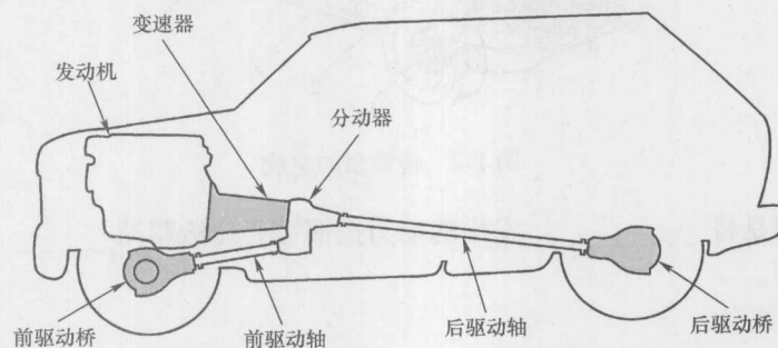
图 1-4 四轮驱动系统
