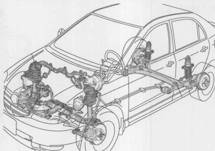
图 1-8 发动机前置前轮驱动
