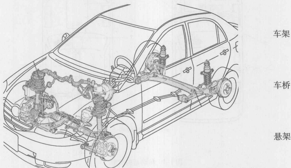
图 1-5 行驶系的组成
