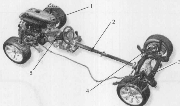
图 1-1 汽车底盘组成
