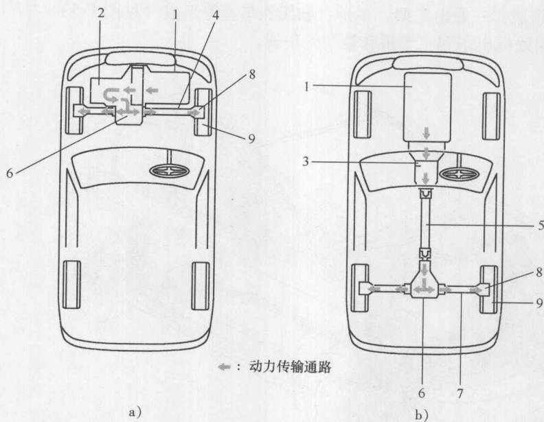
图 1-3 传动系的类型
