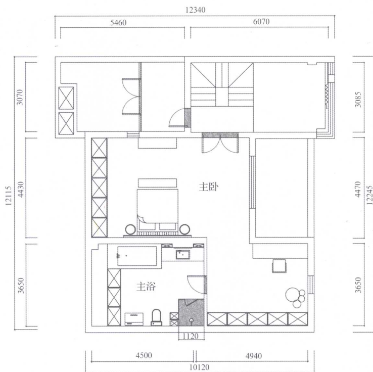
二层平面布置图
