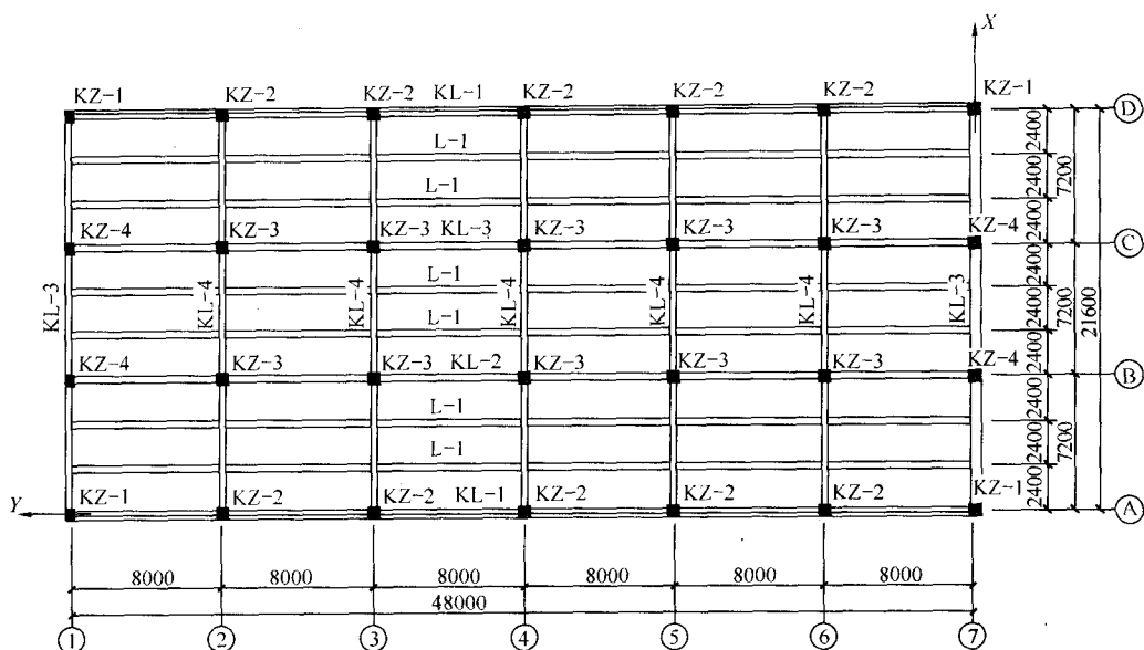
图 1-9-1 结构平面布置图
