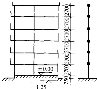
图 1-39-1 剖面图
