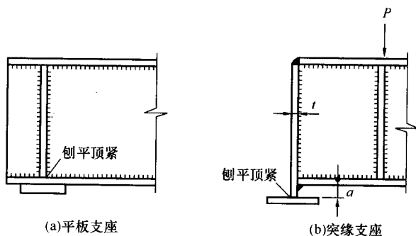
图 1-20-1 梁的支承加劲肋
