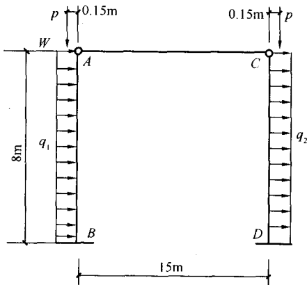
图 1-8-1 排架计算简图
