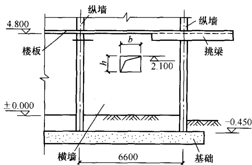
图 1-34-1 底层剖面
