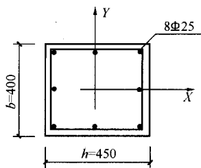
图 1-13-1 柱截面及配筋
