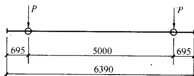
图 1-29-1 吊车轮距及宽度
