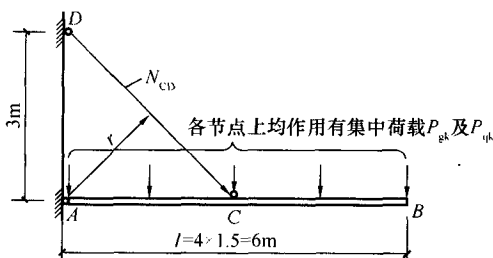
图 1-23-1 钢梁挑篷
