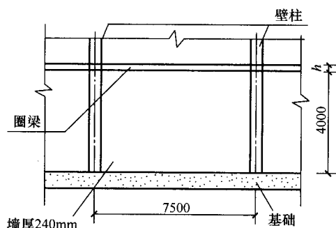
图 1-43-1 外墙立面
