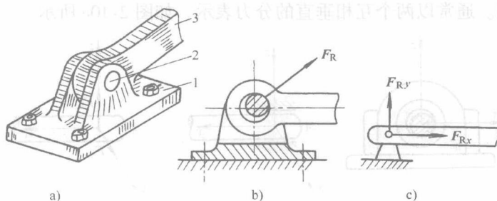
图 2-7 固定铰链支座
