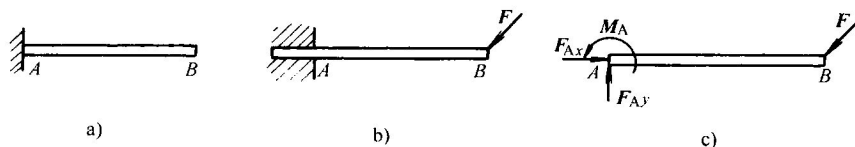
图 2-12 悬臂梁的约束力情况
