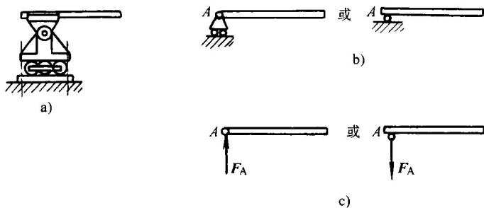
图 2-8 活动铰链支座
