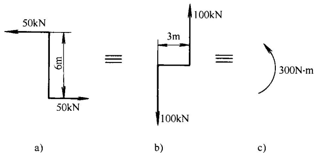
图 2-4 力偶的表示方法
