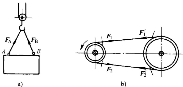
图 2-5 绳索和平带的约束力
