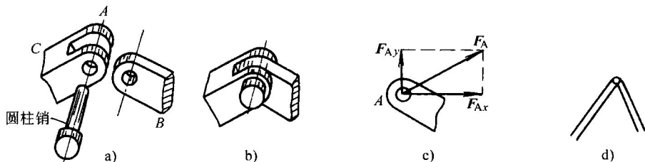
图 2-9 中间铰
