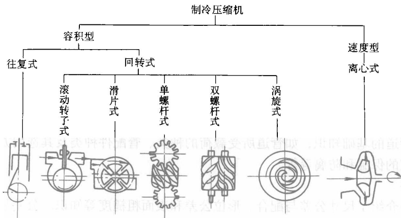
图 1-3 制冷压缩机的分类
