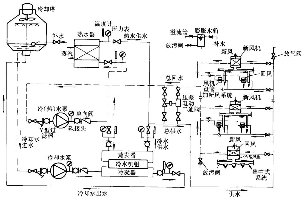
图 1-2 中央空调水系统示意图
