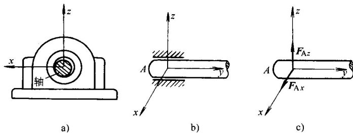
图 2-10 滑动轴承示意图和约束力图
