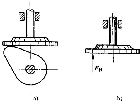
图 2-6 凸轮曲面的约束力
