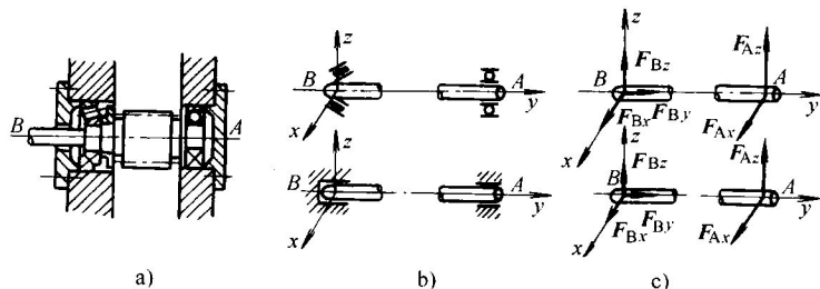
图 2-11 滚动轴承示意图和约束力图
