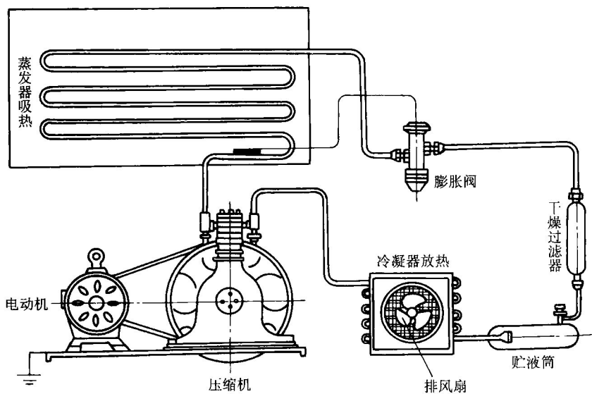
图 1-1 制冷循环
