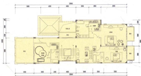
二层平面图
