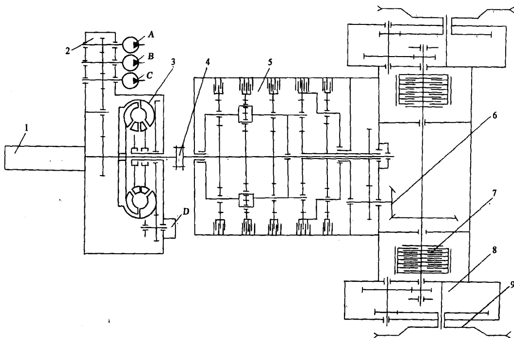
图 1-2b) 推土机液力-机械式传动系布置简图
