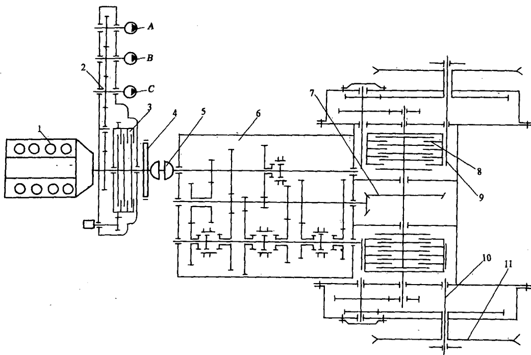
图 1-2a) TY180 履带推土机传动系布置简图
