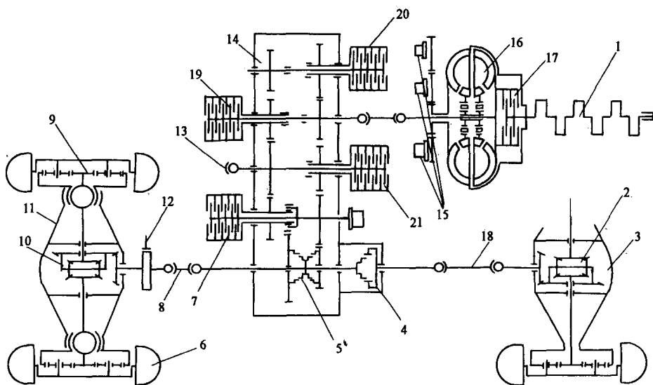
图 1-3 TL160 轮式推土机传动系
