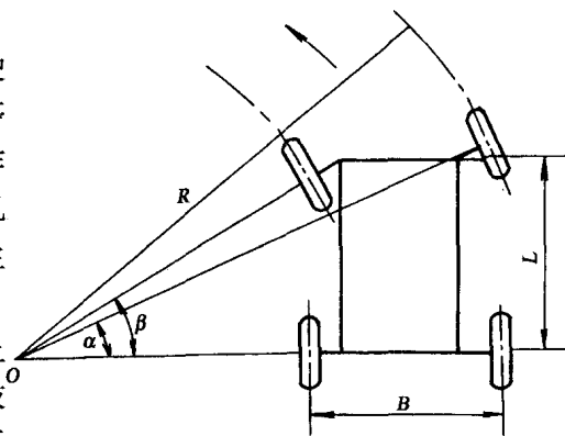
图 1-4 偏转车轮转向方式的示意图
