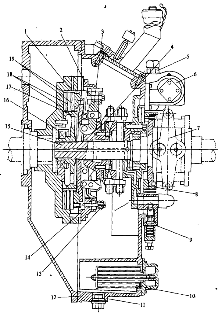
图 1-5 上海 TY320(D150A)推土机的多片湿式主离合器
