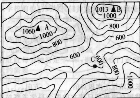
等高线地形图(单位:米)
