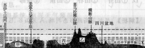
亚洲大陆沿北纬30度的地形剖面图
