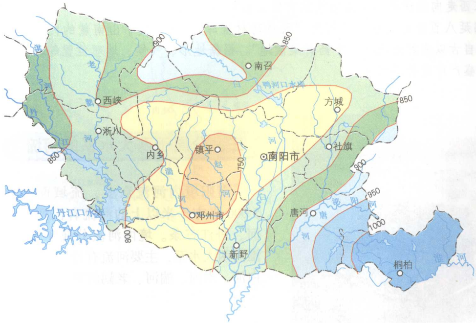
图 2-5 南阳年降水量分布
