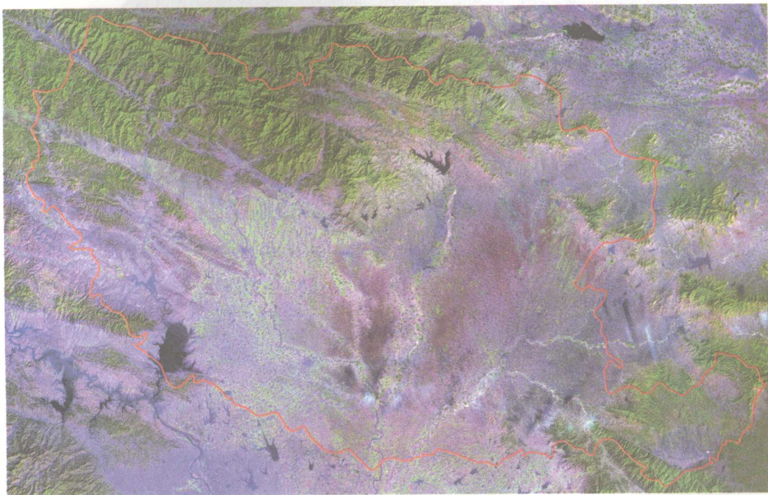
图 2-2 南阳卫星照片
