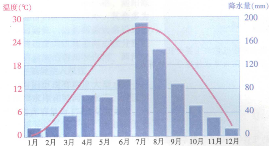
图 2-4 南阳月平均气温和降水量变化示意
