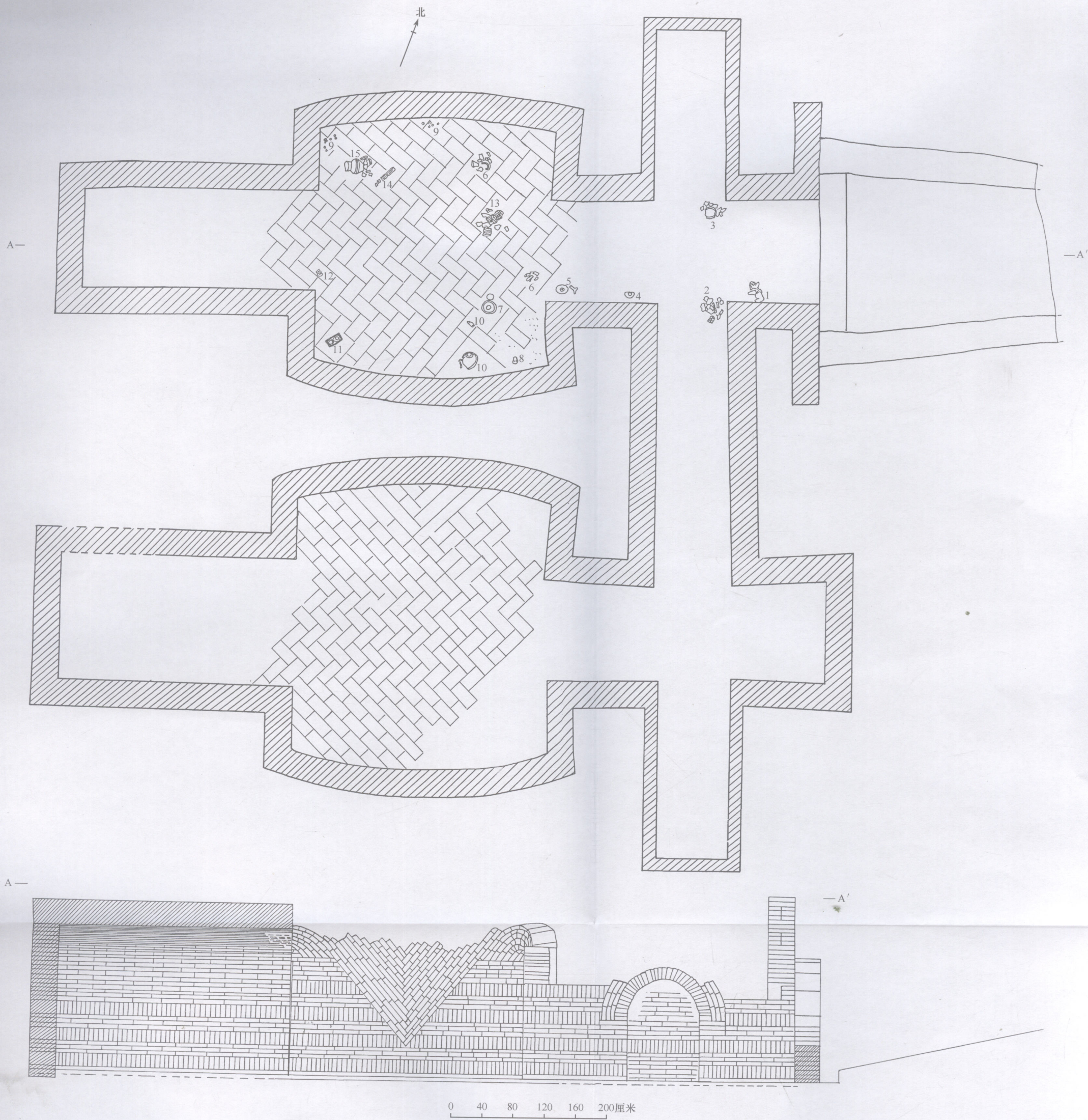
图二九 M8 平、剖面图
