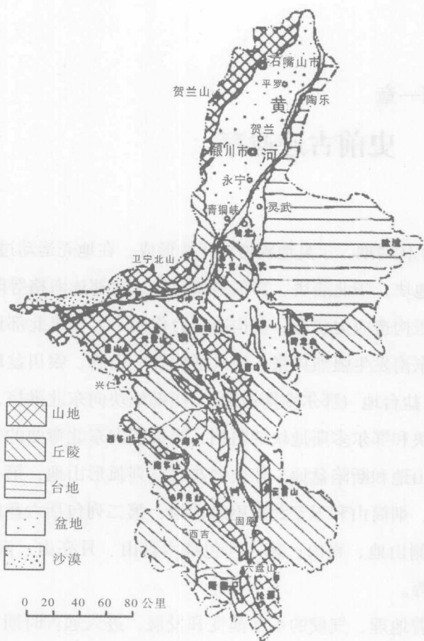
宁夏回族自治区地貌略图
