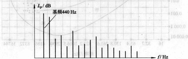
图1-1 钢琴的频谱
