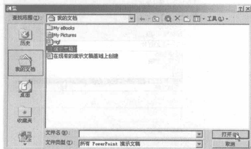
图 1.7 “浏览”对话框
