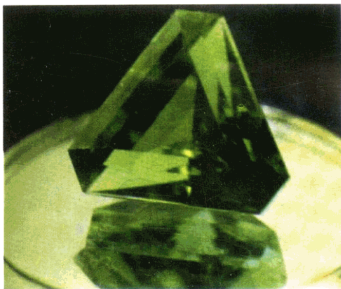
▲ 橄榄石
