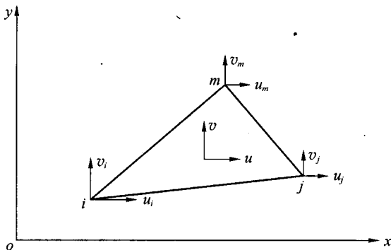
图 2-1 三结点三角形单元
