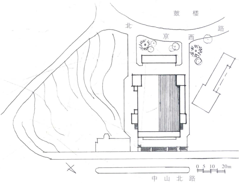
总平面
