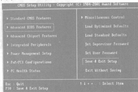
图 1-1 BIOS 主界面
