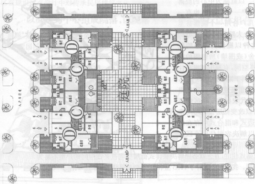
图 1-5(b) 厦门市西柯镇潘塗小区的院落组织 (二)
