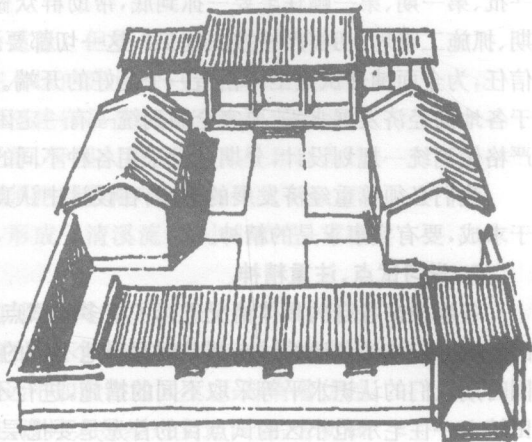
图 1-1(b) 北京小型四合院
