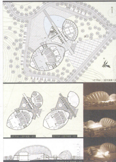
OPERA HOUSE DESIGN OF SHENZHEN UNIVERSITY 深圳大学多功能会演中心建筑设计 功能图 C
