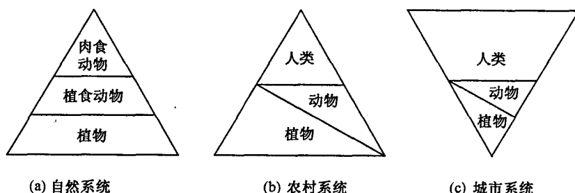
图 1.2 不同类型生态系统的营养结构
